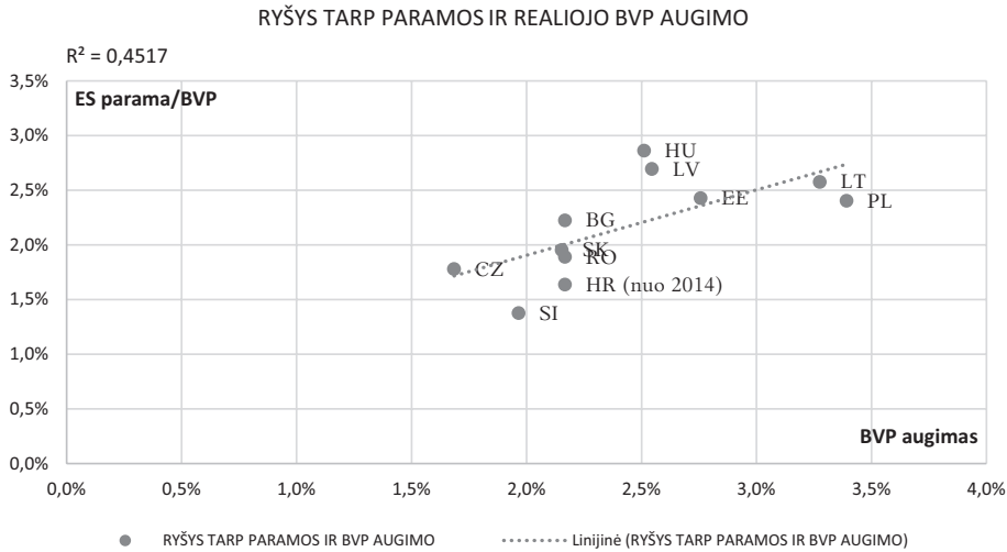
4 pav. 2 lentelės duomenys, pateikti XY grafiko formatu.
